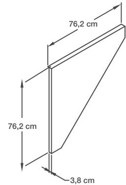
Figura 1 — Dimensiones 6KWL6
