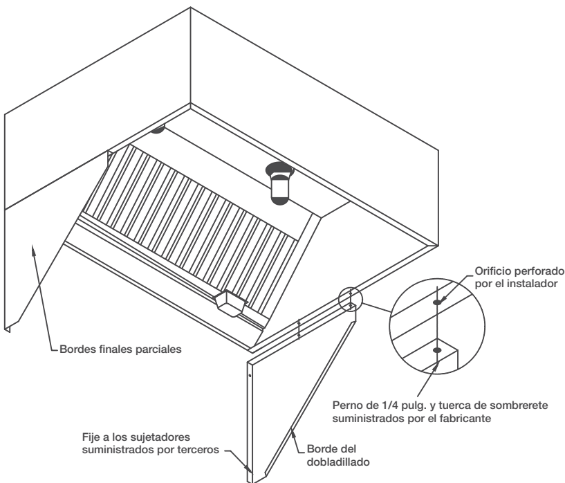
Figura 2 — Instalación Típica
